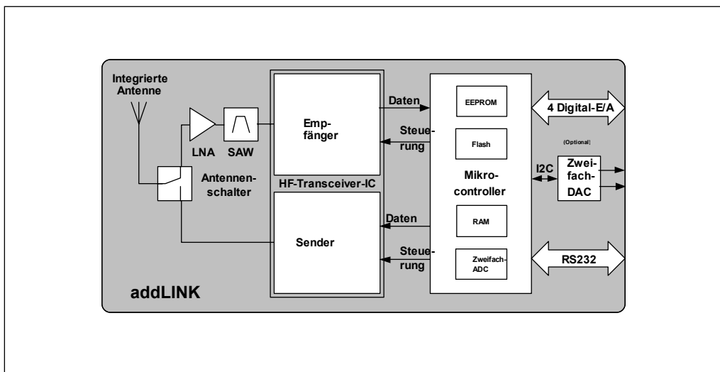
Abbildung 1-1: addLINK-Blockschaubild
