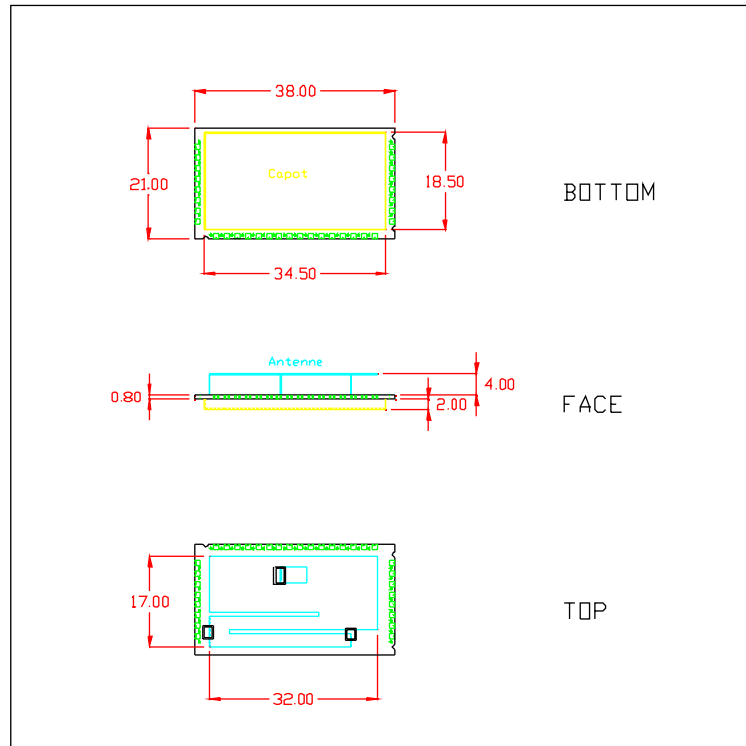
Abbildung 4-2: addLINK-Maße
